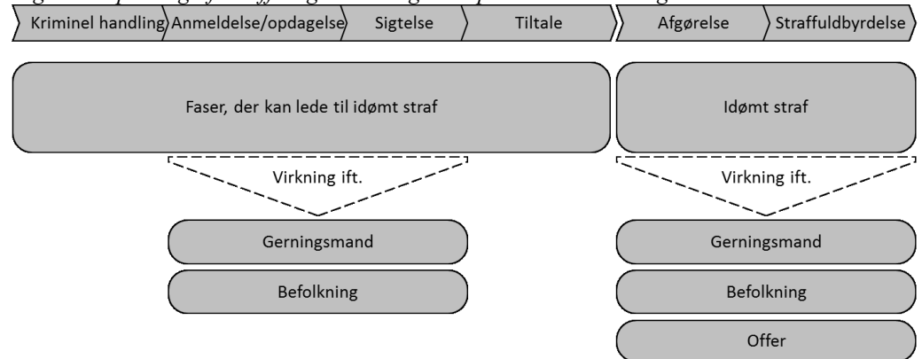
Figur 1: Opdeling af straffesagskæden og dens potentielle virkninger.
