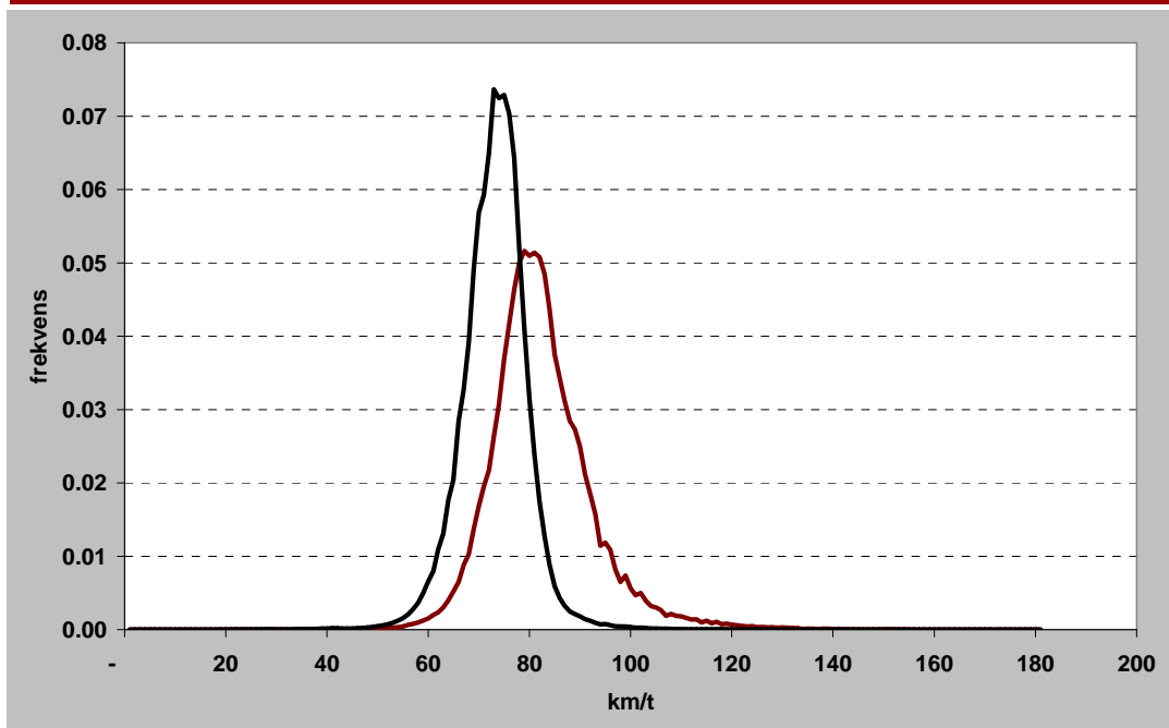
Figur 2.5 Frekvensfordeling af hastigheder før opsætning af ATK (rødbrun) og efter opsætning (sort)
